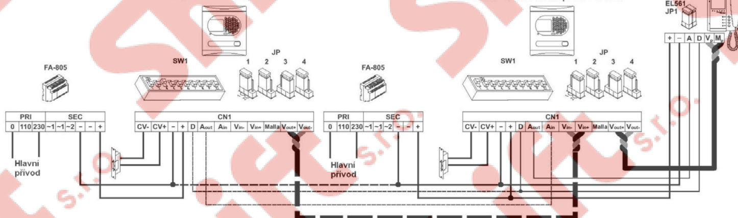
Hlavní - master dveřní panel s videem
